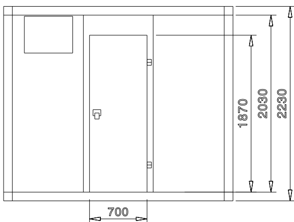
Zij aanzicht
